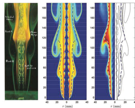
Flujo alrededor de una llama
