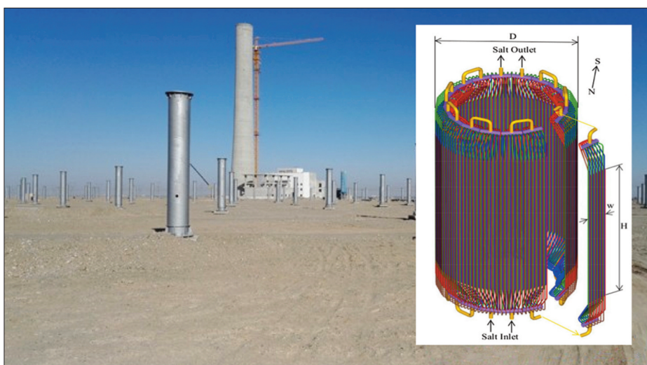
Receptor central de sales diseñado por el grupo ISE del IGM para la central termosolar en construcción de Dunhuang en China
